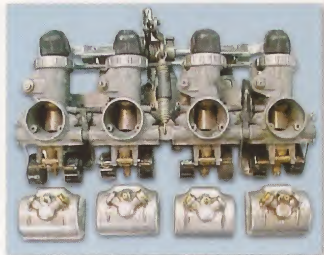
Batería de carburadores de alta cilindrada
